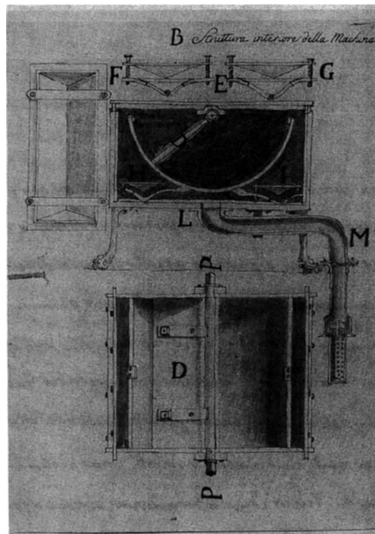
Disegno acquerellato della struttura interna di un «idroballo» ossia di una macchina da utilizzare per il sollevamento delle acque (allegato alla dissertazione di Agostino Litta, poi pubblicata, del 1780, n. 45/16).
