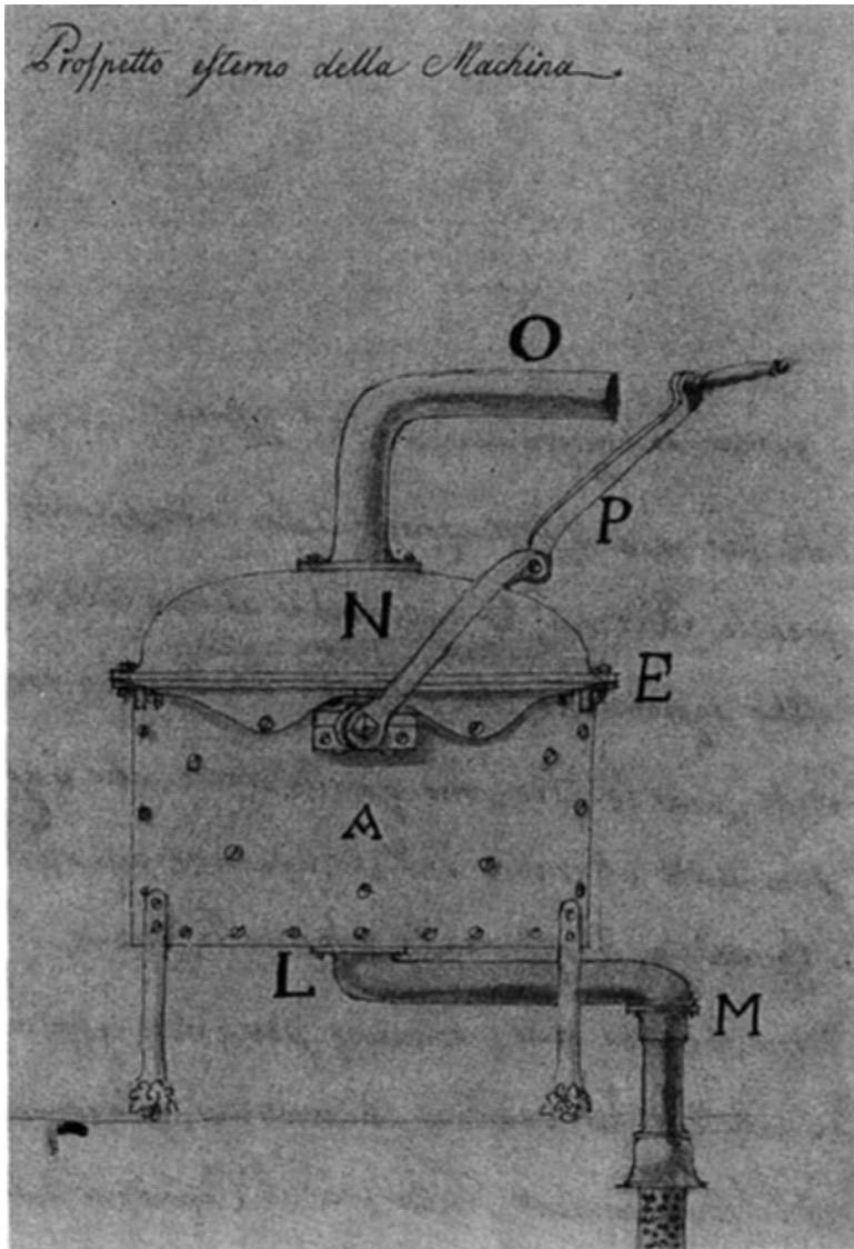
Disegno acquerellato dell'esterno dell'«idrobalò» (dissertazione n. 45/16).
