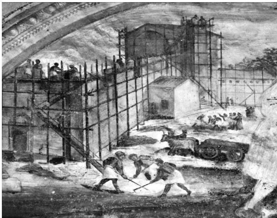
Fig. 2 - Curtatone (Mantova), Santuario della Beata Vergine, affresco nel sottoportico frontale. Cantiere per edificio in muratura . Sono riconoscibili muratori all'opera sui ponteggi, braccianti intenti al trasporto dei materiali e, in primo piano, 'maltaroli' impegnati nell'impasto della calce.
